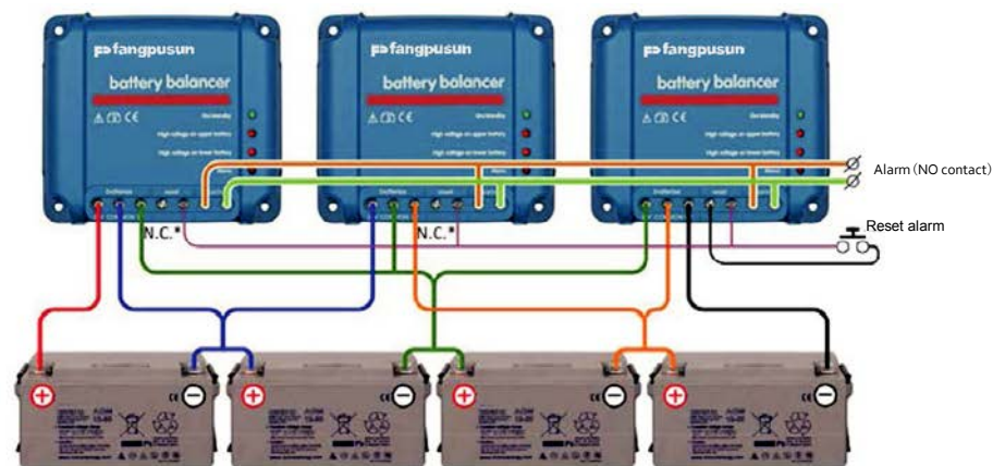
Три акумуляторні балансирі підключені до чотирьох послідовно з'єднаних батарей 12В (система 48В)
