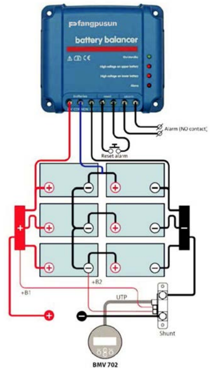
Балансир акумулятора, підключений до шести послідовно з'єднаних 12В батарей (система 24В)
